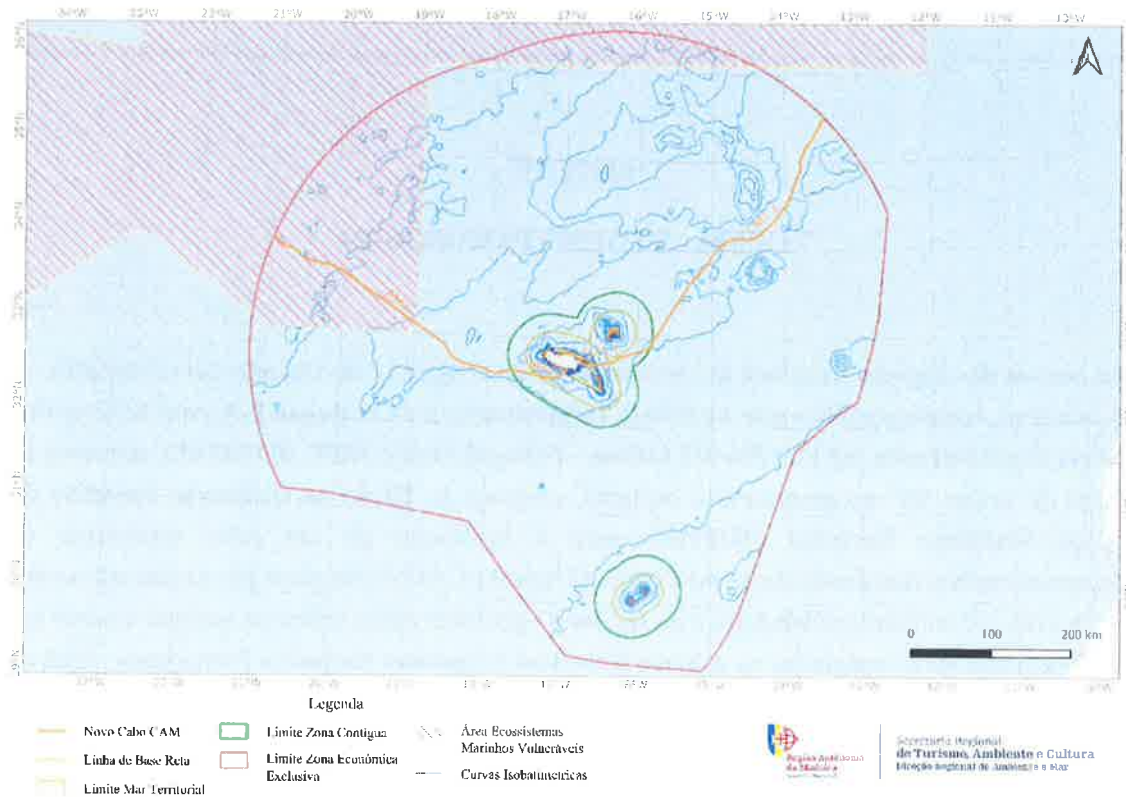
Figura 1. Traçado geral do cabo submarino Atlantic CAM.
