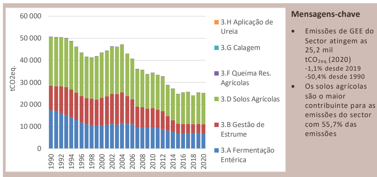
Figura 24: Evolução das Emissões do Sector Agricultura
