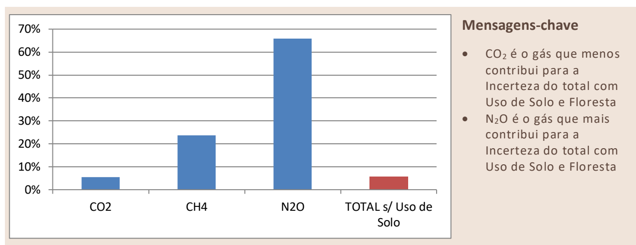
Figura 78: Distribuição da Incerteza Com Uso de Solo por Gás de Efeito de Estufa em 2020
