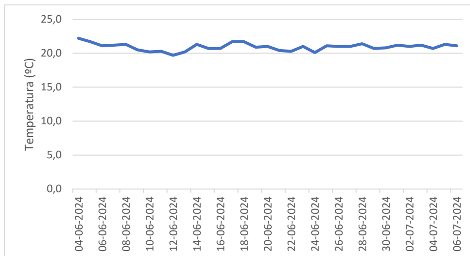
Figura 14 Temperatura.
