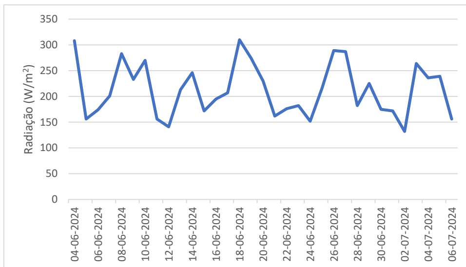
Figura 12 – Radiação solar.
