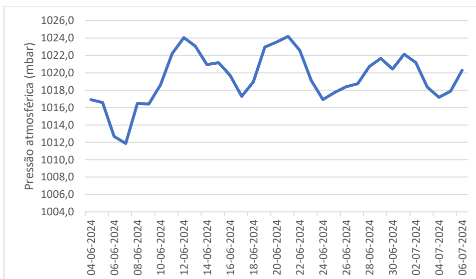
Figura 15 Pressão atmosférica.
