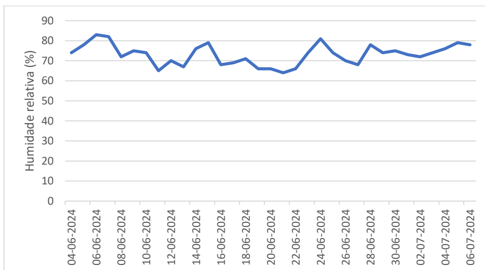
Figura 13 – Humidade relativa.
