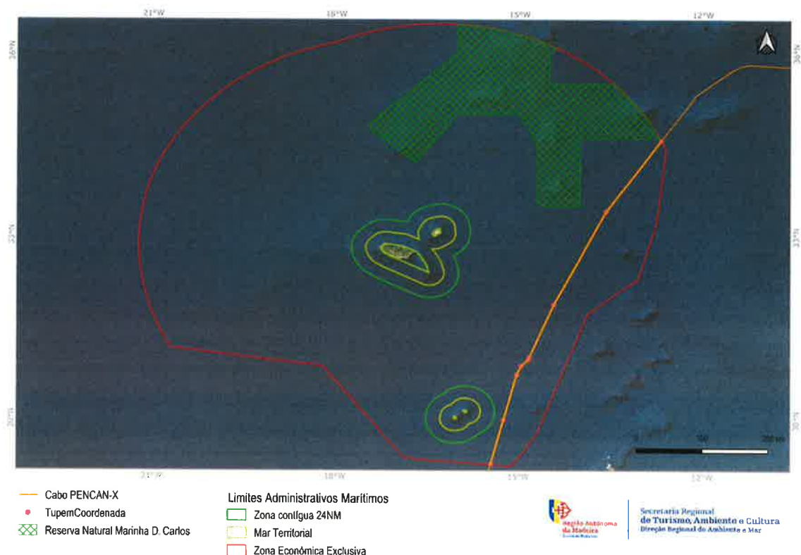
Figura 1. Traçado geral do cabo submarino PENCAN-X .
