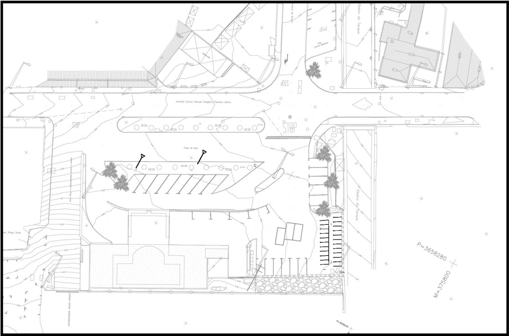
PLANTA DO EXISTENTE ESC.1/500
